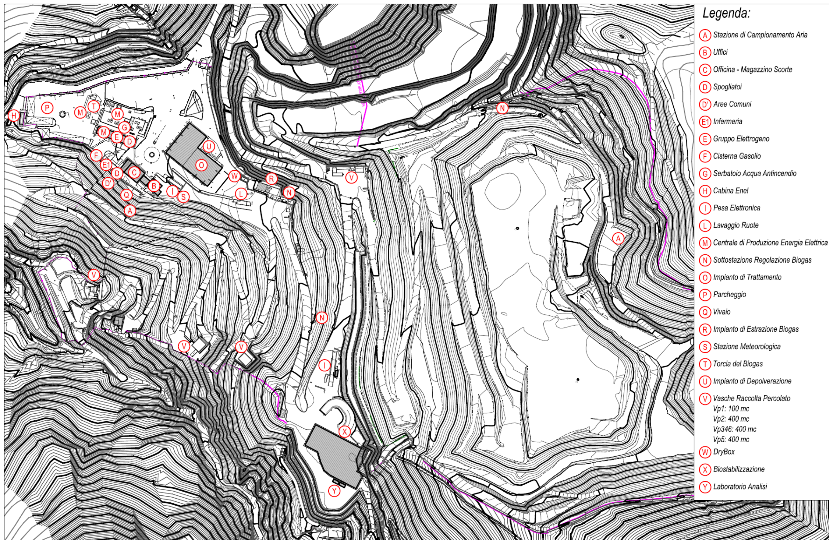
Tav 1: Impianto del Boscaccio - Planimetria Stato Attuale Scala 1:2000
